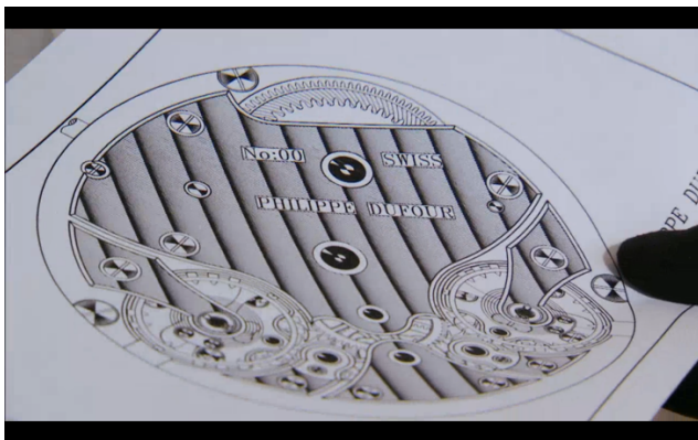
Montre Philippe Dufour à deux balanciers
