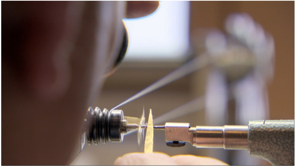
Adoucissage au fer (en laiton) de d'une pièce entre-pointe avec entraineur.
